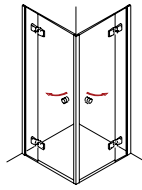
KENOS 220 EckEinstieg mit 2 Drehtüren an Fixteilen
