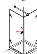
PENDO 130 Pendeltür mit Seiten- wand
