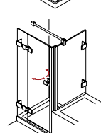
PENDO 231 Pendeltür am Fixteil mit verkürzter Seiten- wand
