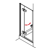
HEIDRA PLAN 200 Drehtür am Fixteil in Nische
