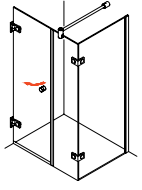
KENOS 140 Drehtür und Fixteil mit Seitenwand
