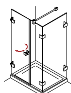
PENDO 140 Pendeltür und Fixteil mit Seitenwand
