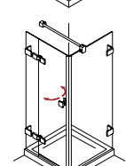
PENDO 230 Pendeltür am Fixteil mit Seitenwand
